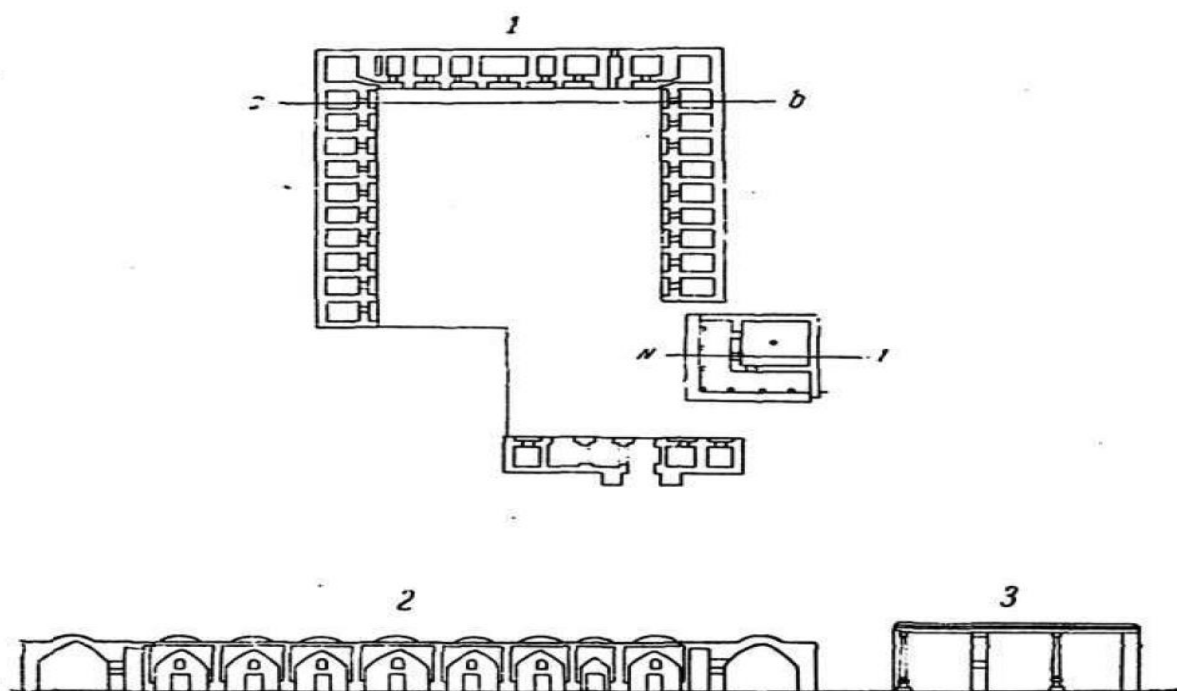
Shayboniyxon madrasasi. Reja va kesimlar (1871-yildagi). 1.Madrasa rejasi. 2.A–B chizig'i bo'yicha fasad. 3.chizig'i bo'yicha kesim. Manba: R.G. Muqminovning “К истории аграрных отношений в Узбекистане XVI в. По материалам «Вакф-наме».
